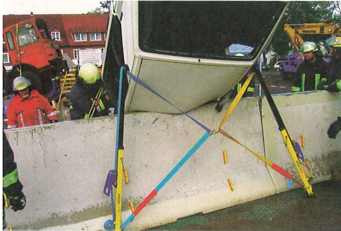
Mit dem Stabilisierungssystem StabFast wird das Fahrzeug gesichert.
